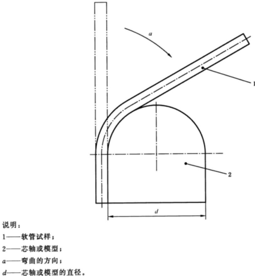
图 3 使用芯轴或模型的试验装置
