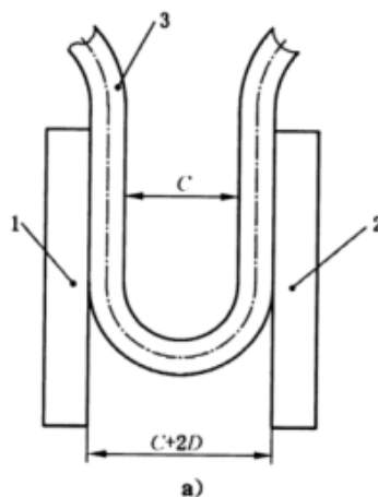
图 1 弯曲试验装置
