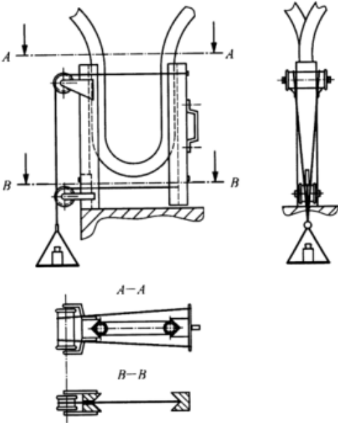
图 2 滑轮和砝码试验装置
